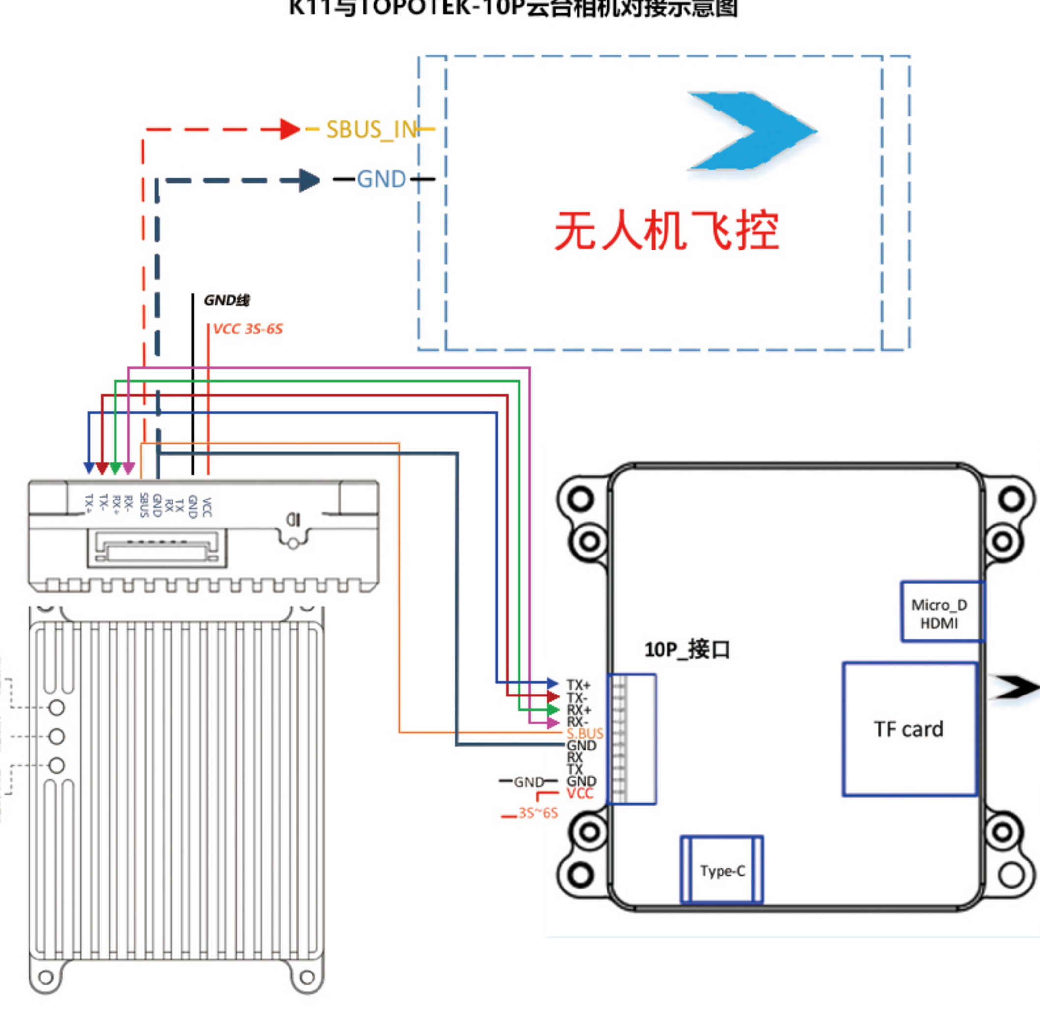
K11与TOPOTEK-10P云台相机对接示意图
