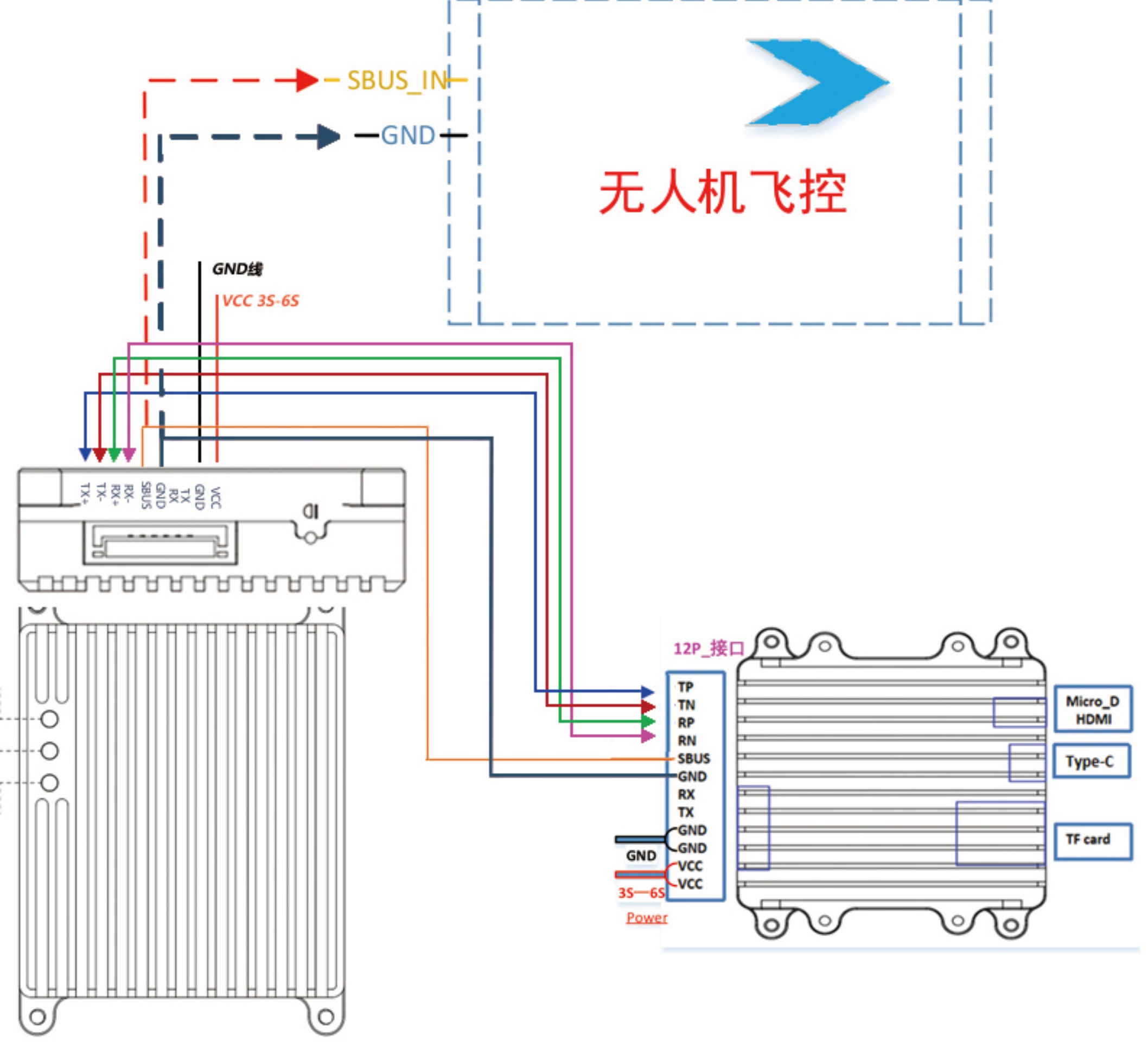
K11与TOPOTEK-12P云台相机对接示意图
